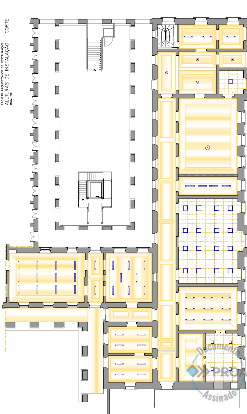
PROJETO ARQUITETÔNICO DE RESTAURAÇÃO LOCAÇÃO DE EQUIPAMENTOS NOS FORROS - 1º PAVIMENTO ESCALA 1:100
