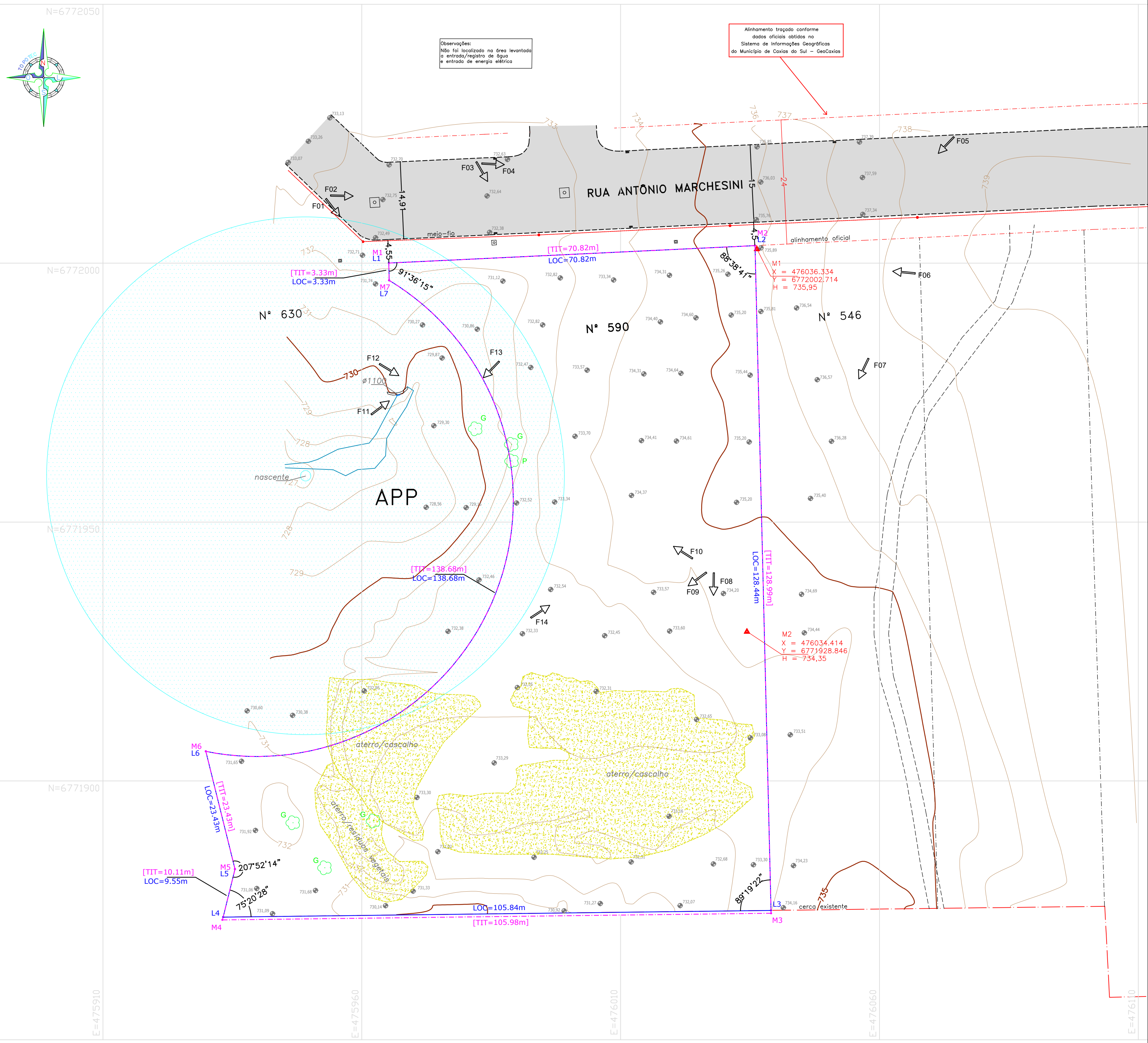
PLANTA DE LOCALIZAÇÃO ESCALA: 1/500
