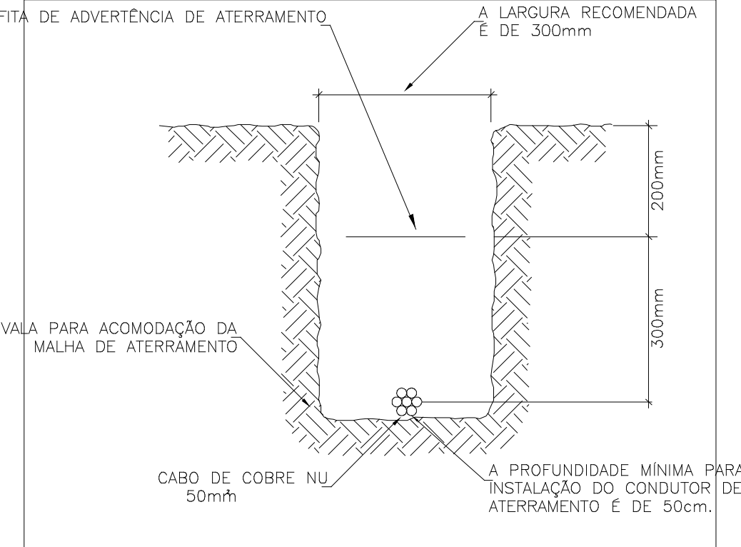
DETALHE 07 - VALA PARA ACOMODÇÃO DA MALHA DE ATERRAMENTO
