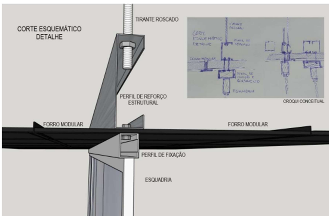
Detalhe esquemático de reforço estrutural e perfil de fixação para esquadria na interface com o forro modular
