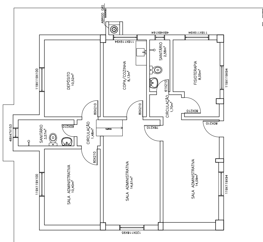
PLANTA BAIXA ESC. 1:50
