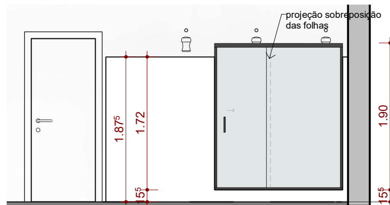
Elevação 8
