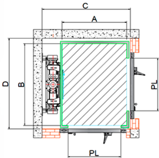
Entradas Adjacentes
