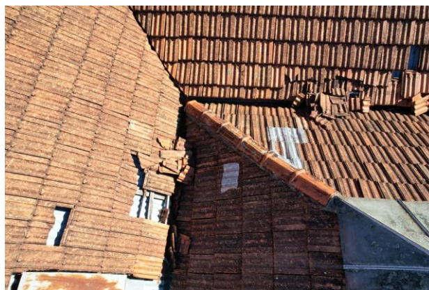
F04 – Vista parcial mostrando a deterioração da cobertura e que abaixo das telhas francesas existem chapas de zinco
