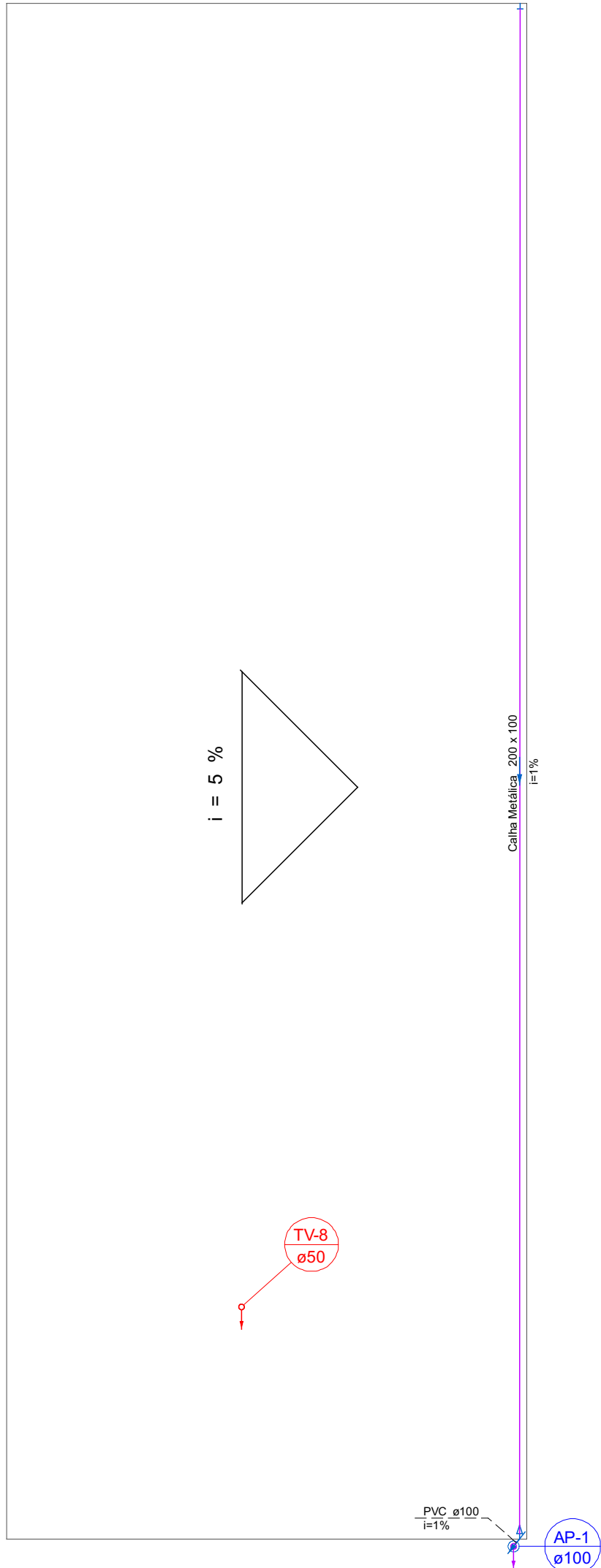
PLANTA COBERTURA - ÁREA TÉCNICA - ESGOTO 1:50
