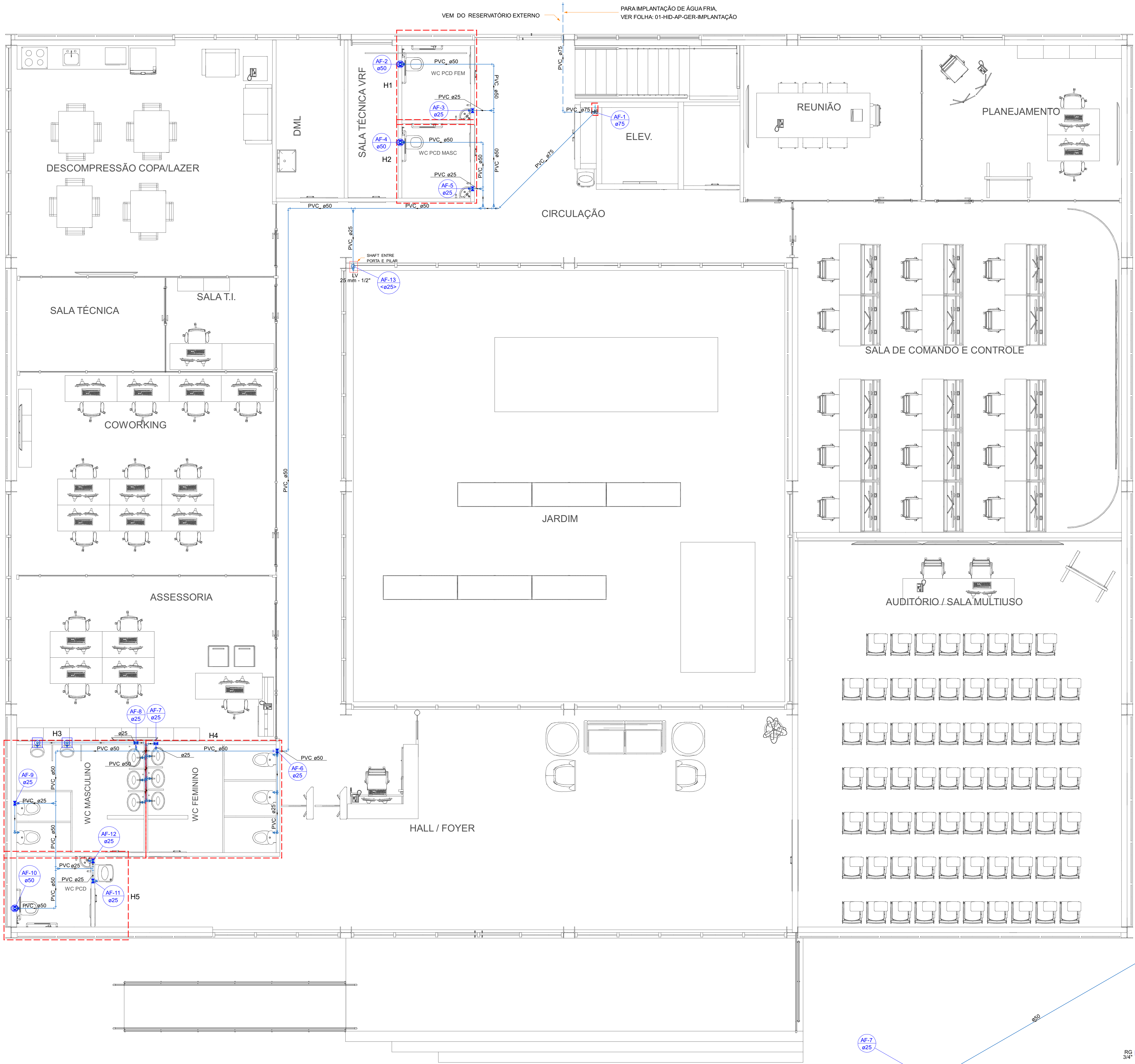
PLANTA BAIXA TERREO - CENTRO DE COMANDO E CONTROLE 1:50
