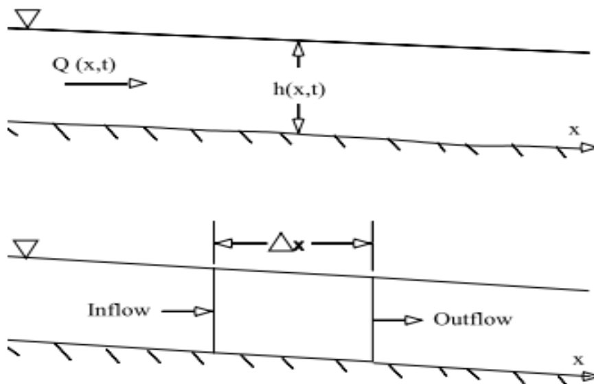
Figura 3 - Volume de controle para derivação da equação da continuidade e momento (Fonte: Consórcio Metroplan Bacia do Rio dos Sinos)
