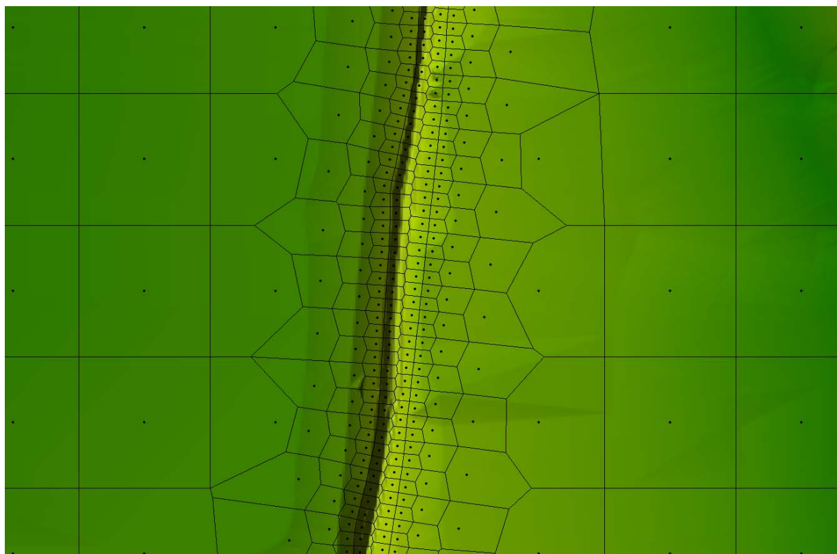
Figura 7 - Exemplo de malha computacional gerada. (Fonte: Consórcio Metroplan Bacia do Rio dos Sinos)
