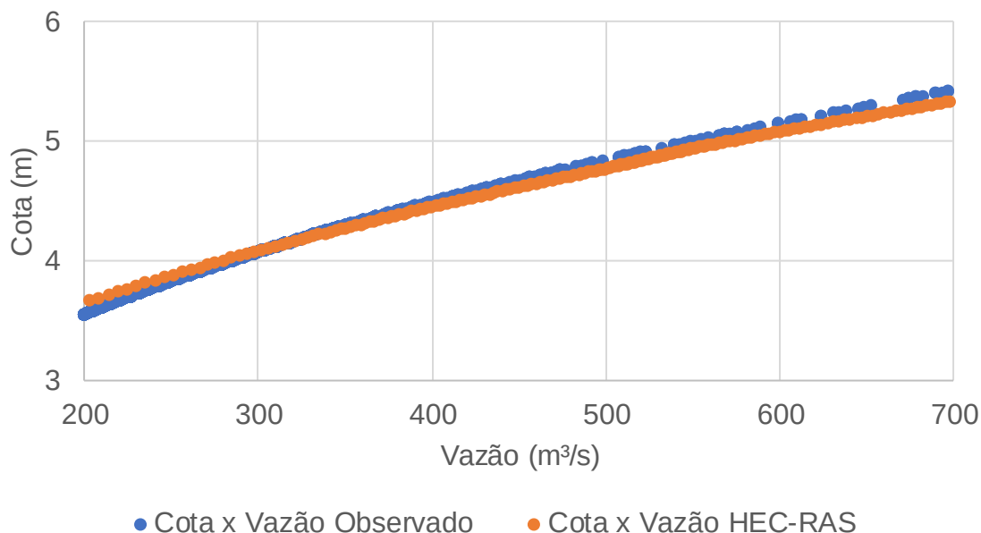
Figura 11 - Calibração dos Parâmetros Hidráulicos para a seção Estação São Leopoldo (Fonte: Consórcio Metroplan Bacia do Rio dos Sinos)
