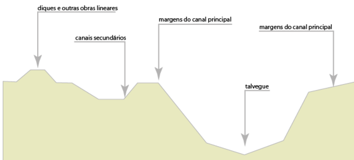
Figura 6 - Elementos principais de elevação para reconstituição da superfície (Fonte: Consórcio Metroplan Bacia do Rio dos Sinos)
