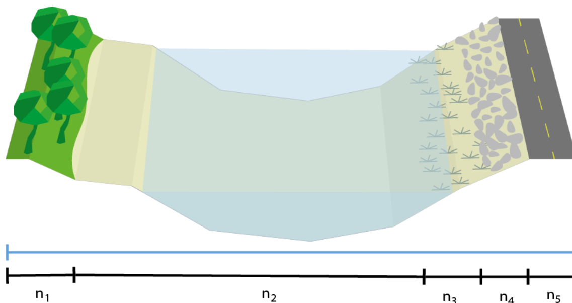
Figura 8 - Exemplo de variação de rugosidade em uma mesma seção hidráulica (Fonte: Consórcio Metroplan Bacia do Rio dos Sinos)
