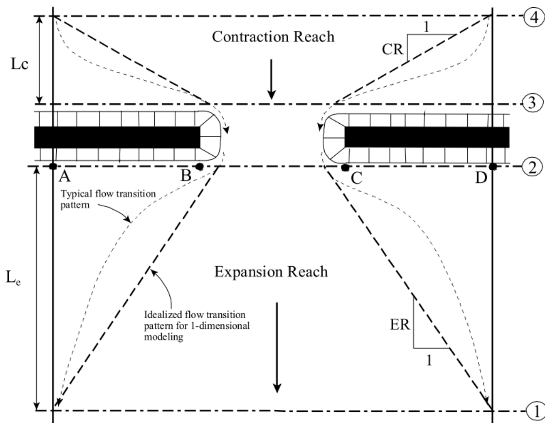
Figura 10 - Seções hidráulicas para representação de uma ponte no HEC-RAS (Fonte: Consórcio Metroplan Bacia do Rio dos Sinos)
