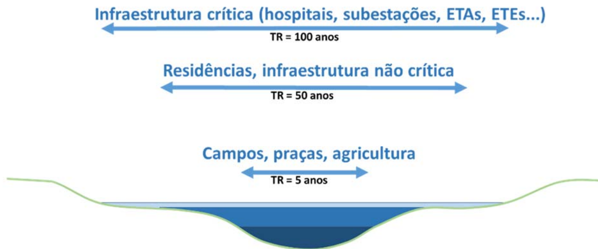
Figura 1 - Potencial ocupação urbana de acordo com o risco associado. (Fonte: Consórcio Metroplan Bacia do Rio dos Sinos)
