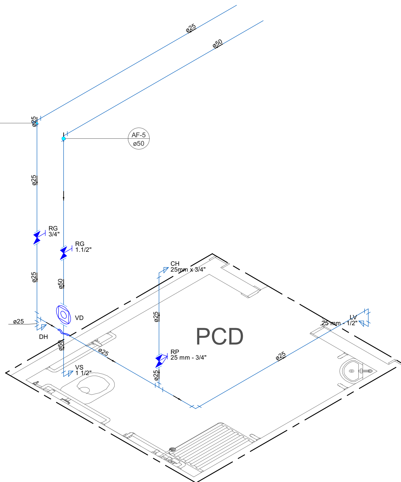
DETALHE H3 1:25
