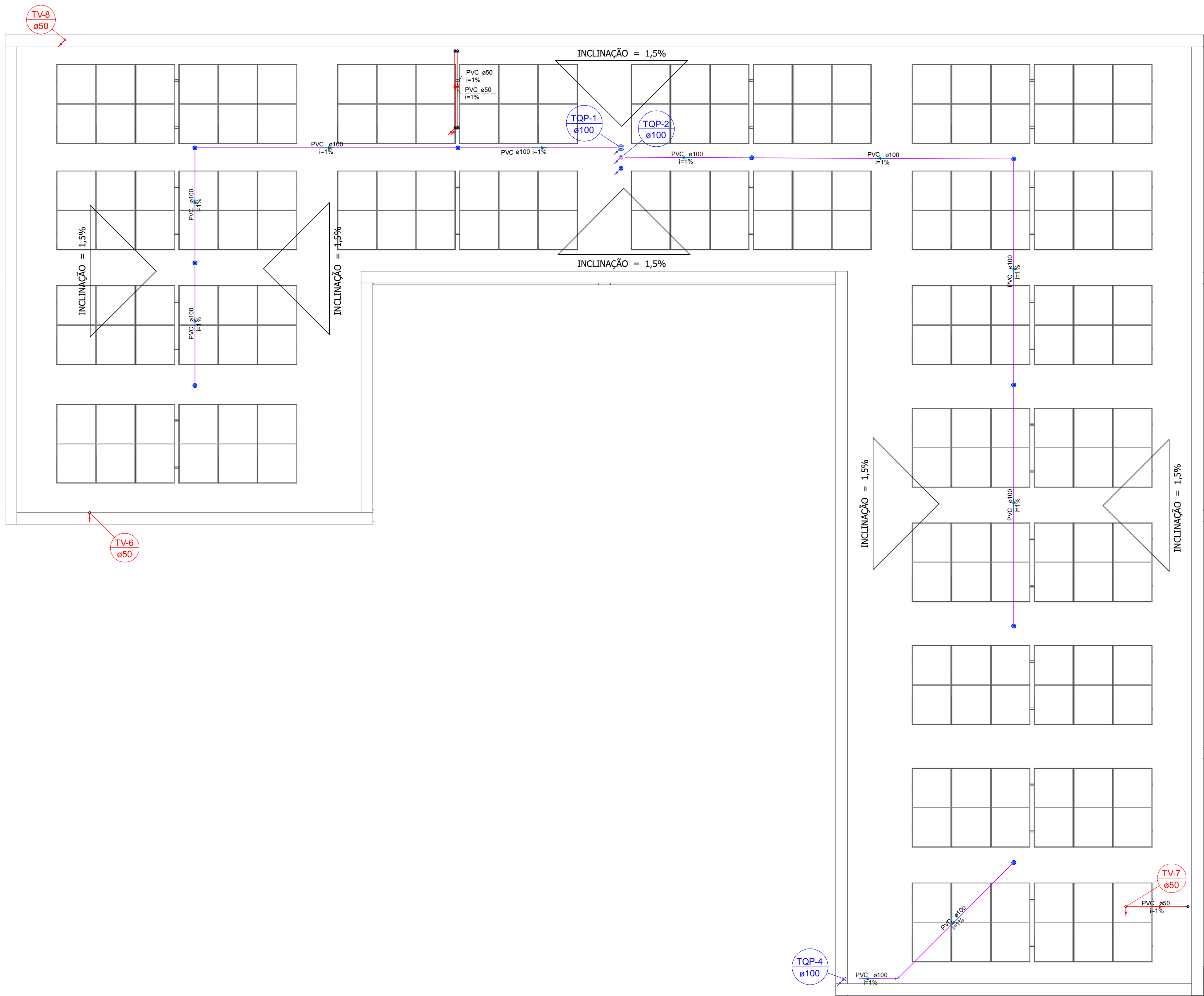
PLANTA BAIXA COBERTURA - CENTRO DE COMANDO E CONTROLE
