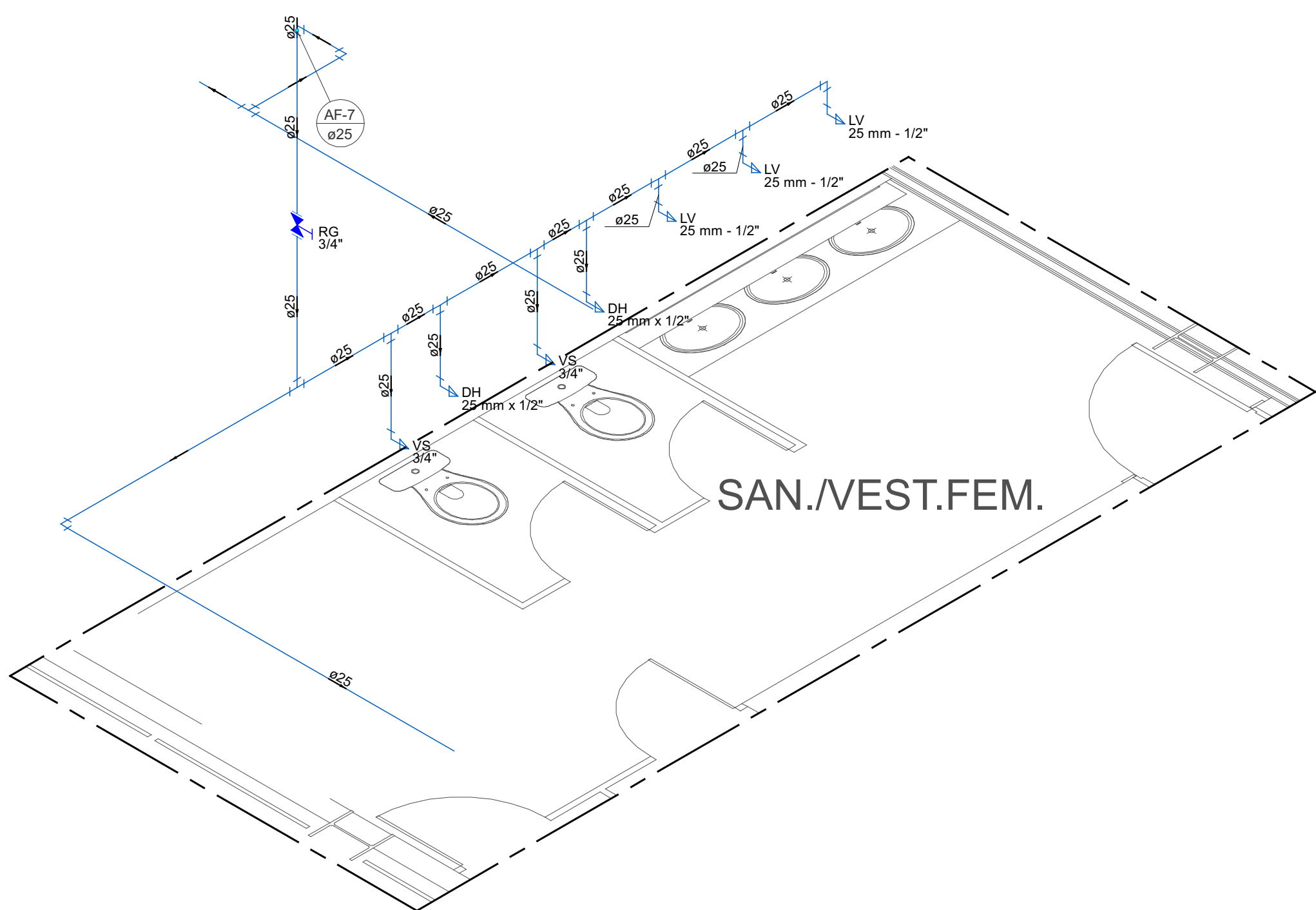
DETALHE H4 1:30
