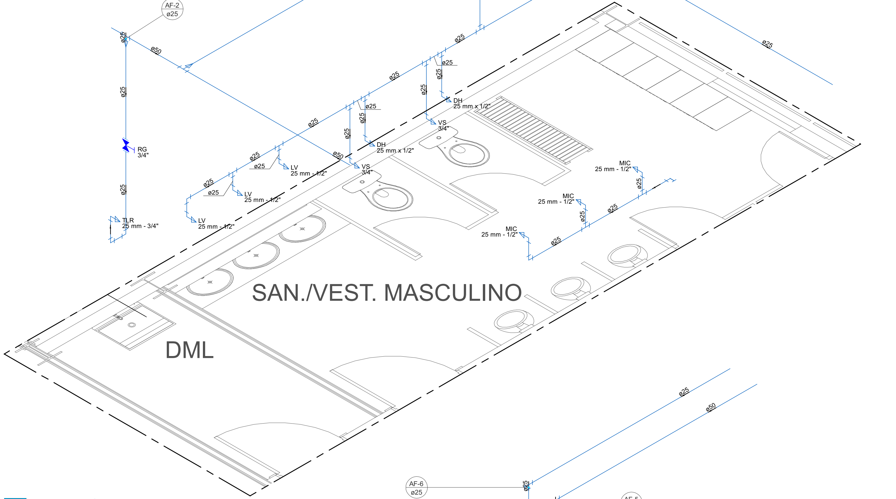
DETALHE H1 1:25
