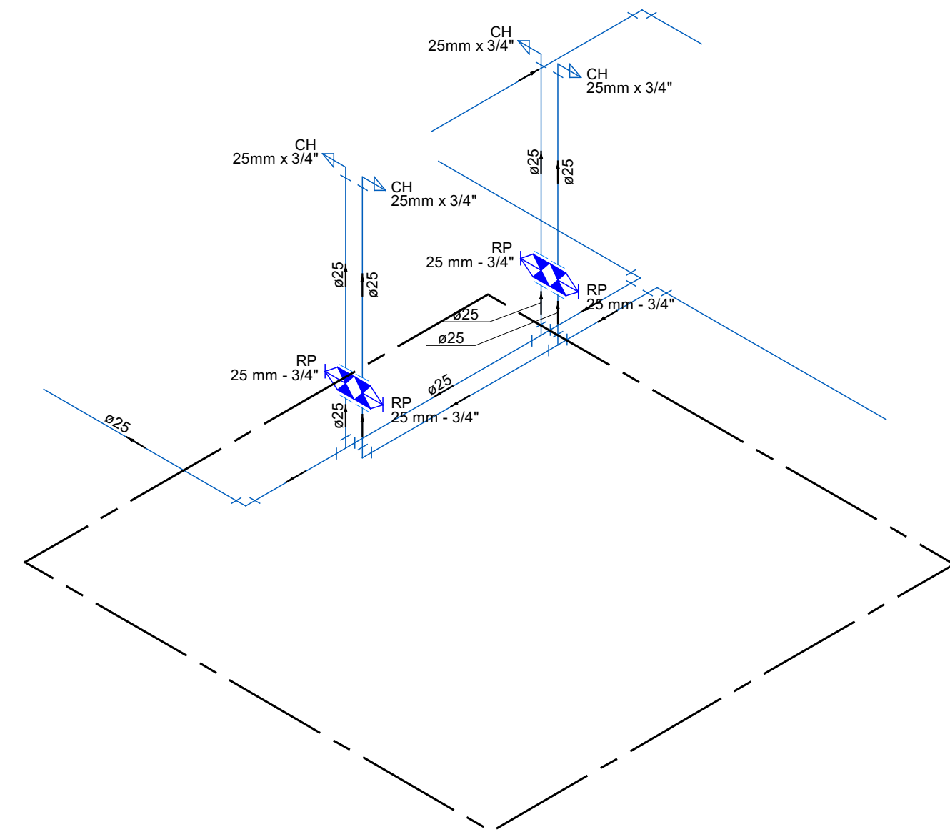
DETALHE H2 1:25
