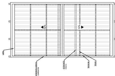
PLANTA BAIXA COBERTURA ESC.: 1/100
