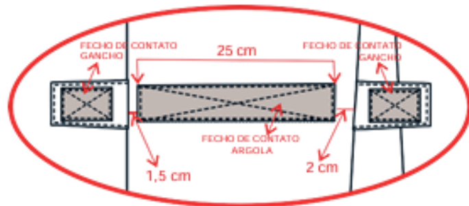
VISÃO DA ALETA DO ENTREPERNAS ESQUERDO (DE QUEM VESTE)
