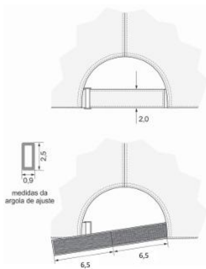
Figura 7 - Detalhes da parte traseira
