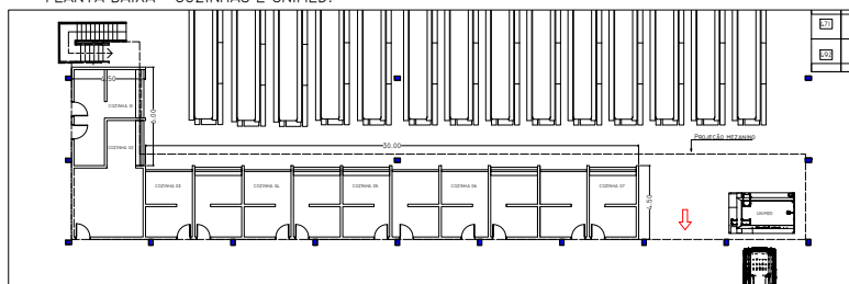
PLANTA BAIXA - COZINHAS E UNIMED.
