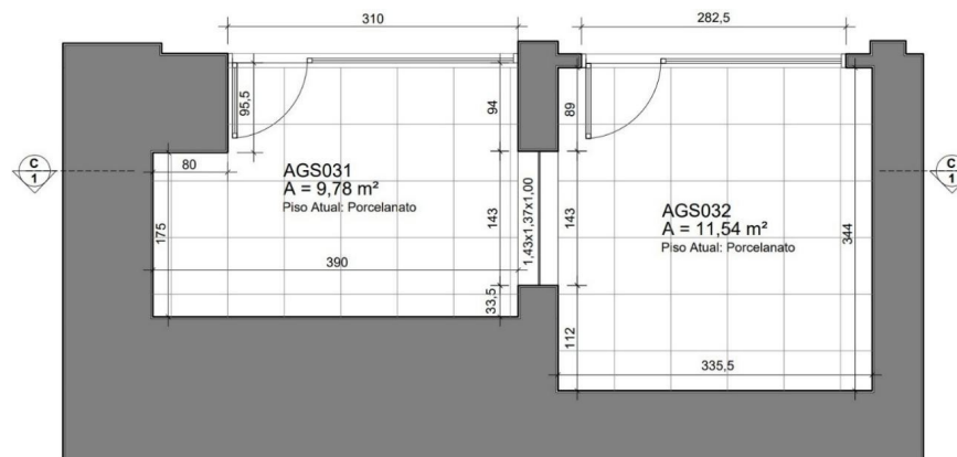
Planta Baixa de Levantamento sem Escala Determinada.
