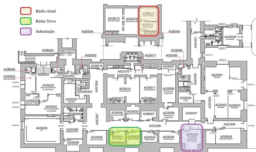
Subsolo Ala Governamental Planta Baixa de Localização - s/esc.
