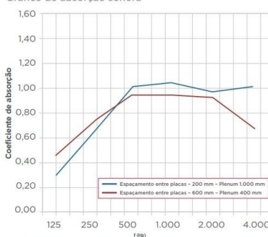
Gráfico de absorção sonora
