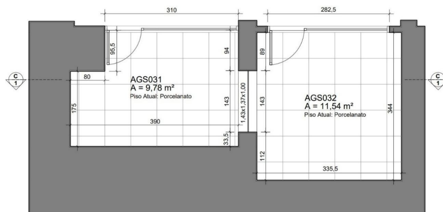
LEVANTAMENTO - PLANTA BAIXA
