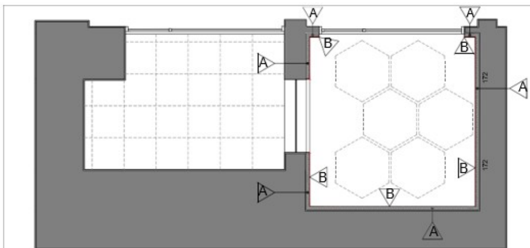
5 PAREDES ACÚSTICA PLANTA BAIXA ESCALA 1:75
