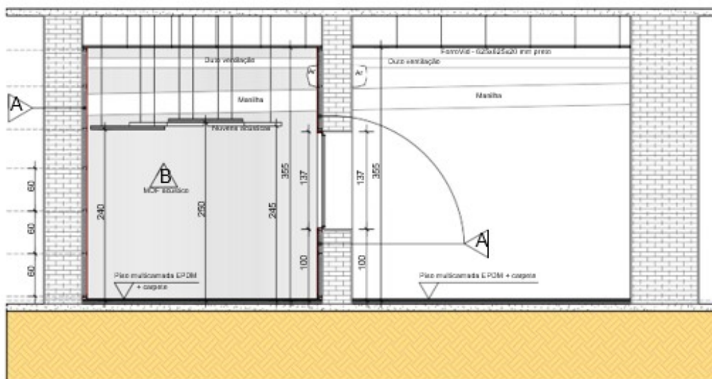
6 PAREDES ACÚSTICA CORTE ESCALA 1:75
