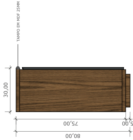
14 VISTA LATERAL ESQUERDA - BALCÃO COFFEE BREAK 1:1,10
