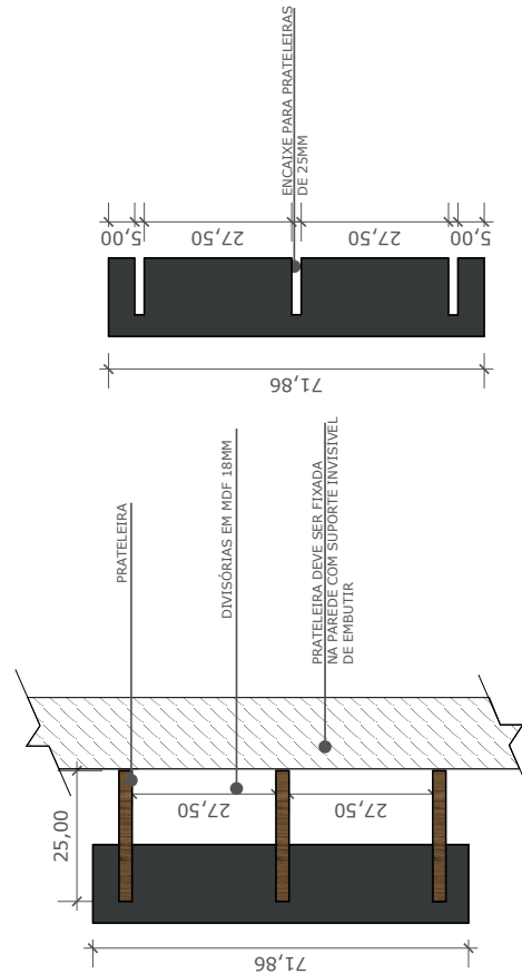
09 VISTA LATERAL ESQUERDA - PRATELEIRA 1:10
