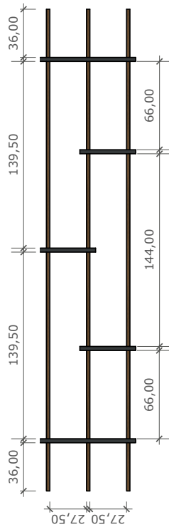
08 VISTA FRONTAL - PRATELEIRA 1:25
