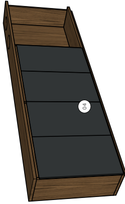
16 ISOMÉTRICA - BALCÃO COFFEE BREAK SEM ESCALA
