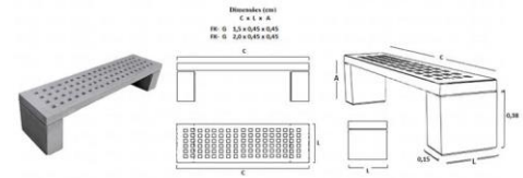
2. Banco em concreto pré-moldado, modelo em grelha
