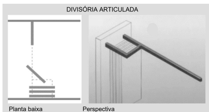
Figura 19 - imagem divisórias articuladas
