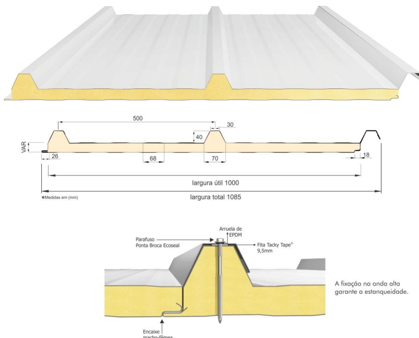
Figura 10 – imagem telha termoacústica
