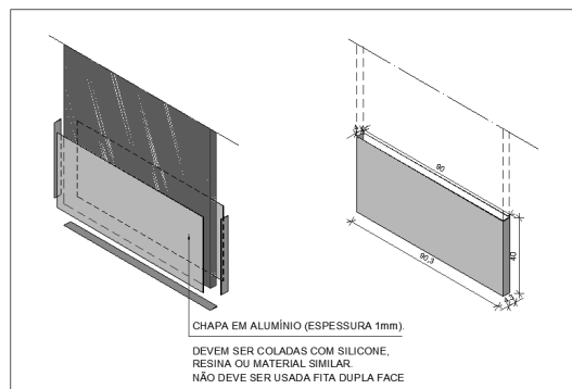
Figura 5 - detalhe chapa metálica para portas de madeira
