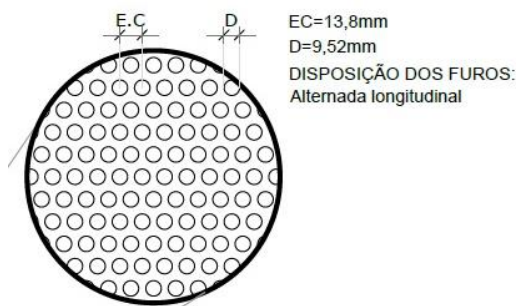
Figura 7 – imagem furos chapa metálica
