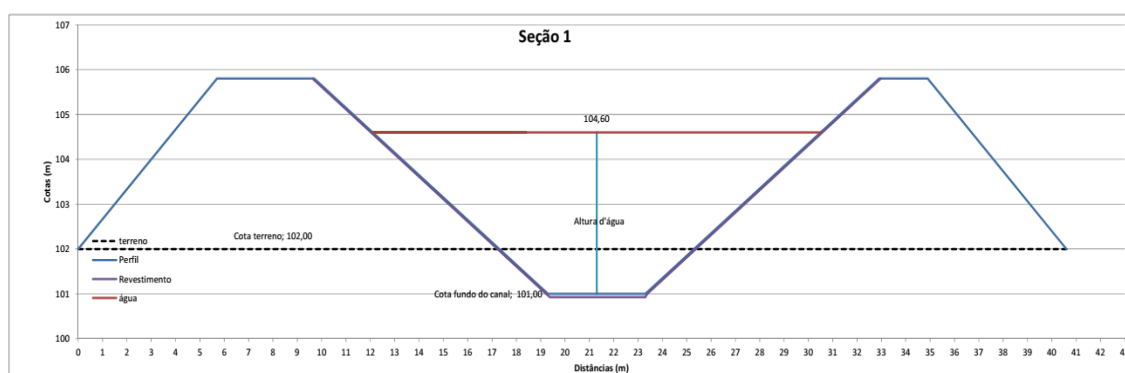
Figura 04 - Canal Secundário Jaguari – Seção tipo 1 - sem revestimento de argila.
