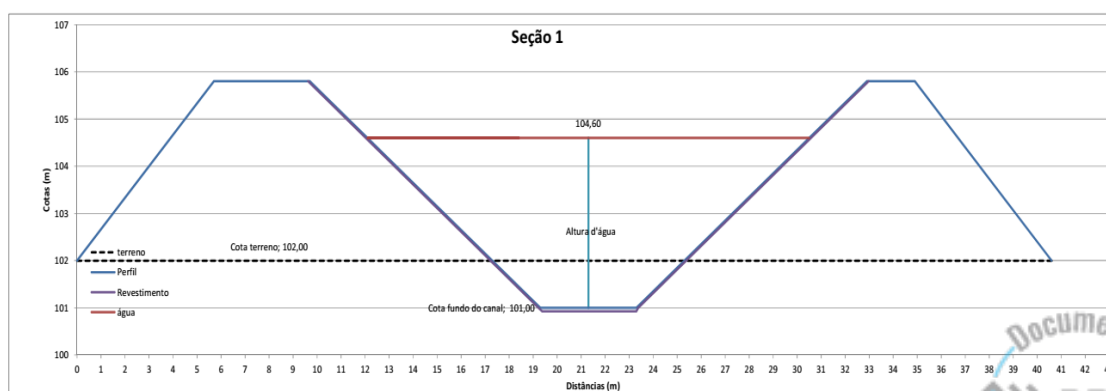
Figura 03 - Canal Principal Jaguari – Seção tipo 1 - sem revestimento de argila.
