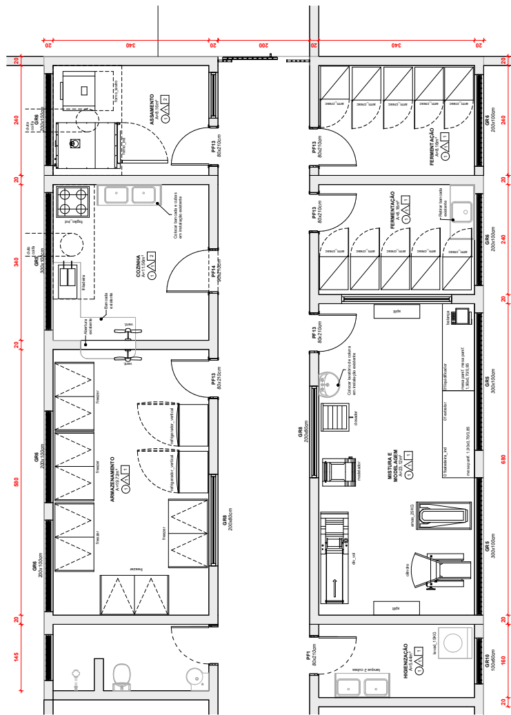
LAYOUT PROCAP PANIFICAÇÃO 1:50
