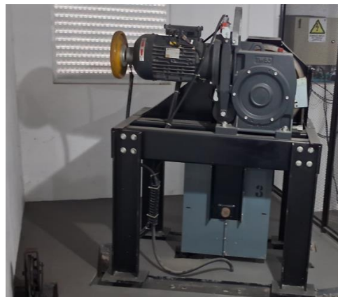
Imagem 11 – Sistema de tração do elevador n° 711 sem proteção.
