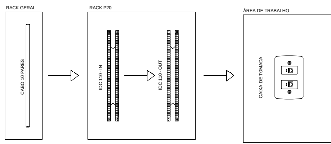
DIAGRAMA DE REDE DE TELEFONIA
