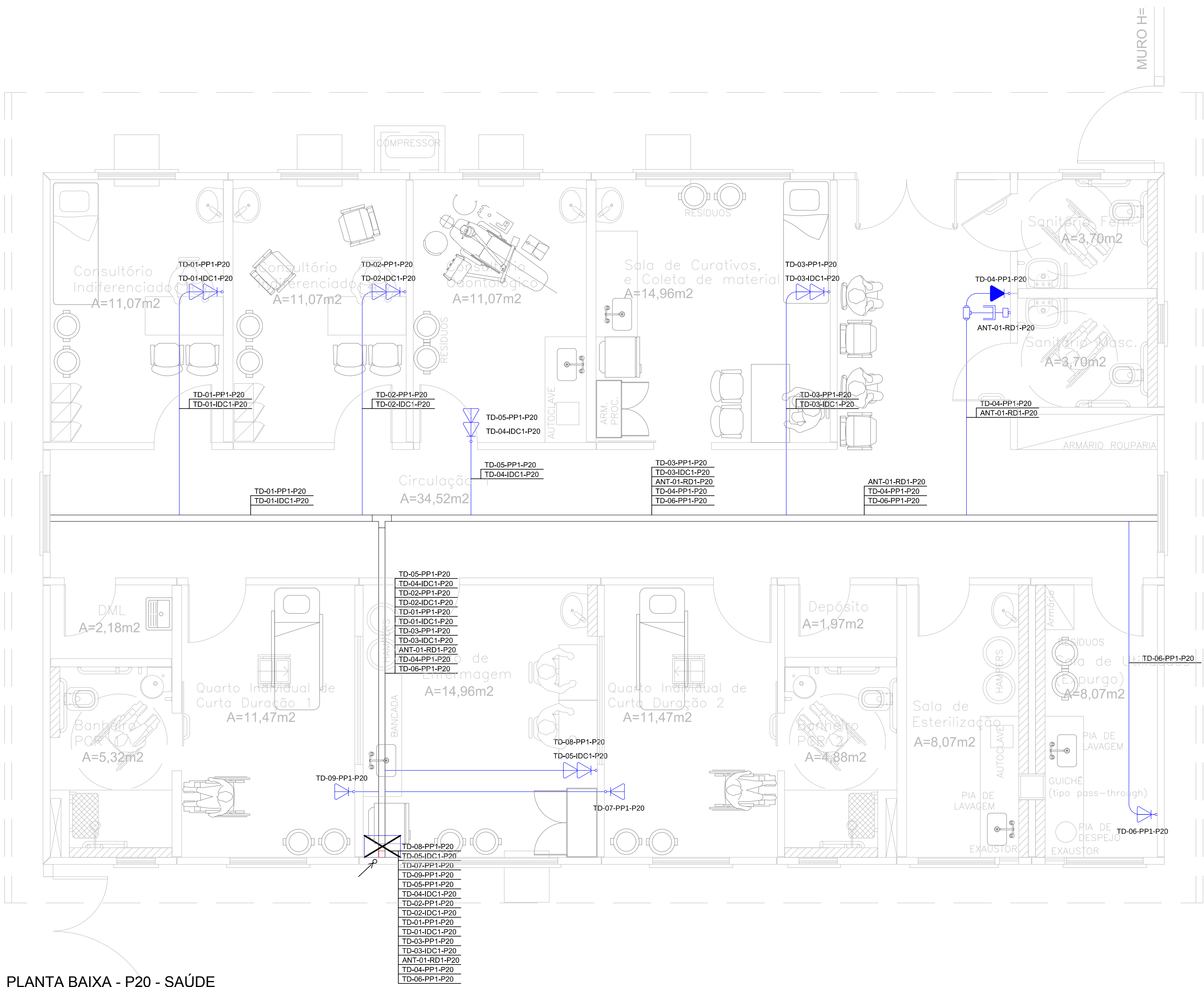
PLANTA BAIXA - P20 - SAÚDE ESCALA 1:50 ÁREA 191,95 m²
