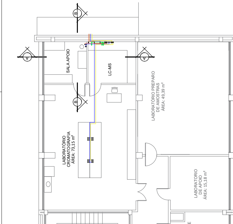
PLANTA BAIXA 4º PAVIMENTO - PRÉDIO 05 LABORATÓRIO DE CROMATOGRAFIA ESCALA 1:50
