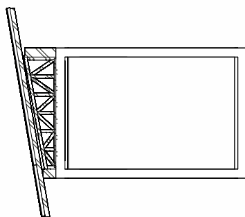
Corte 02 ESC: 1 : 50
