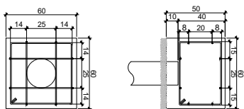
ARMADURA BLOCOS - BL01 (21x) ESC. 1:20
