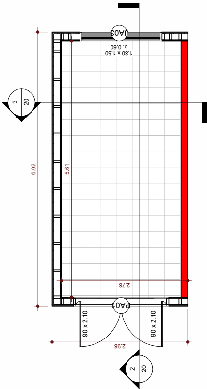
PLANTA BAIXA
