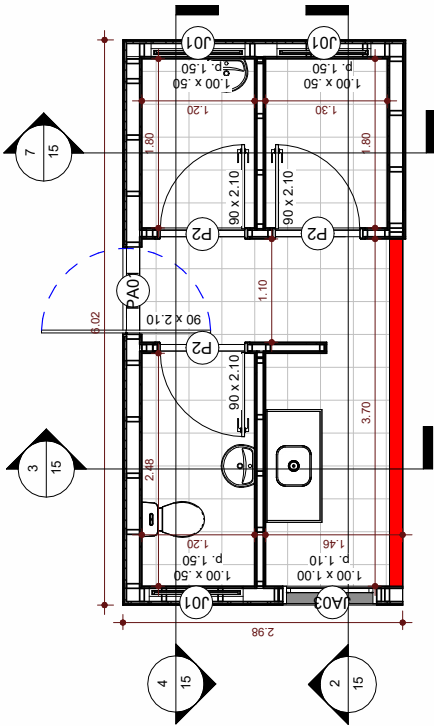
Planta Baixa
