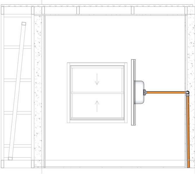
ELE ESG 2 - 02
