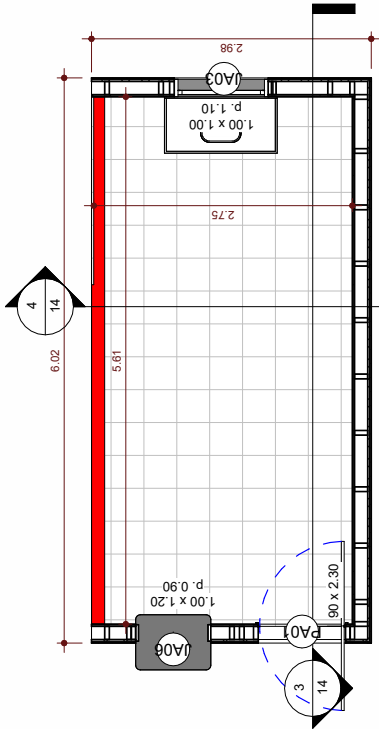
Planta Baixa ESC: 1 : 50
