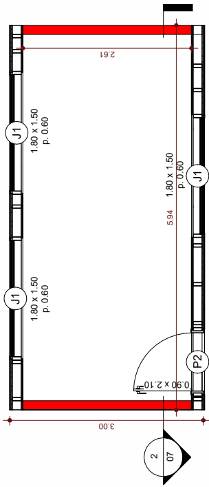
PLANTA BAIXA
