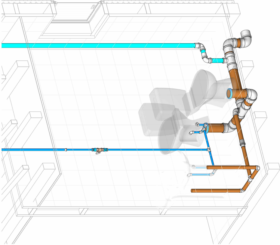
3D COMPATIBILIZAÇÃO
