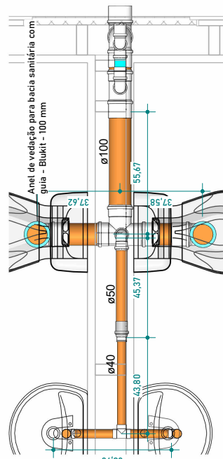
Planta ESG - detalhe 1
