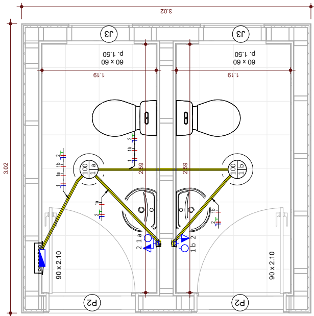
Planta Baixa - Elétrica
