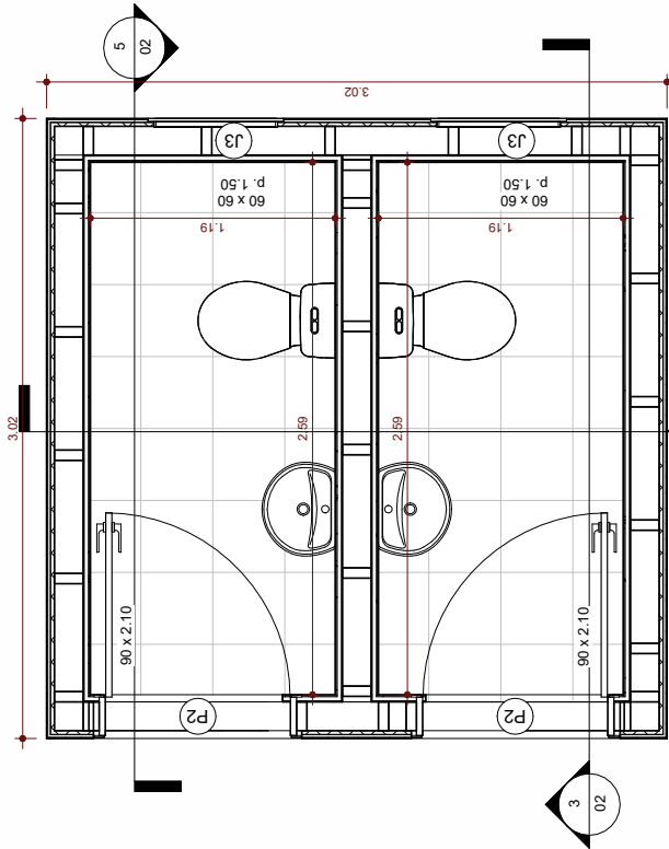
PLANTA BAIXA ESC: 1 : 25
