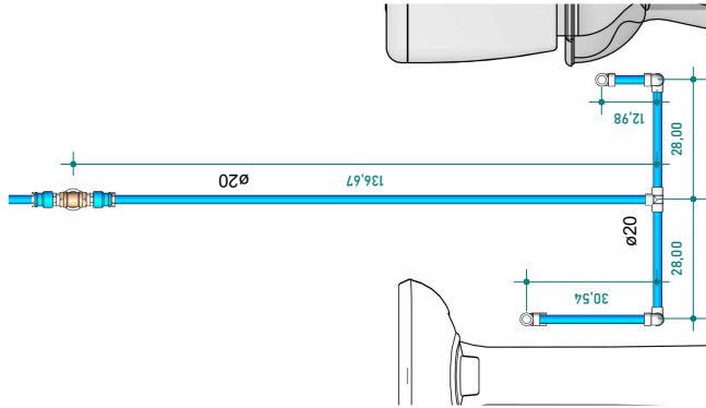
Detalhe HID - 02
