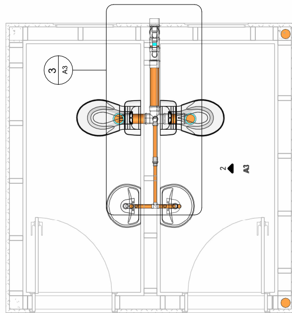
Planta ESG
