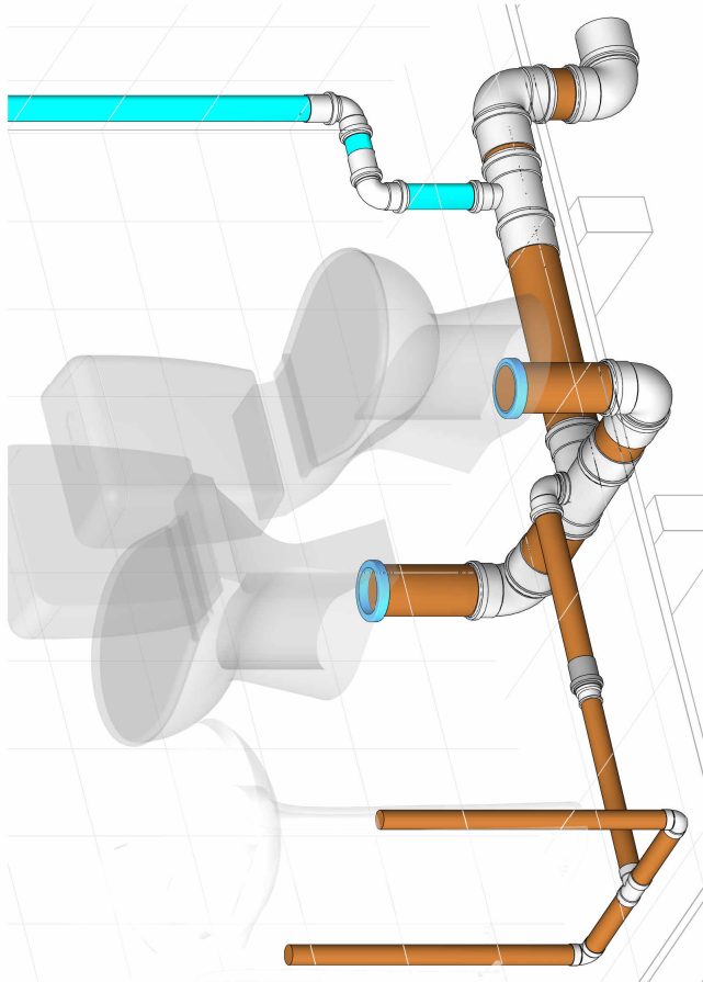
3D ESG Detalhe
