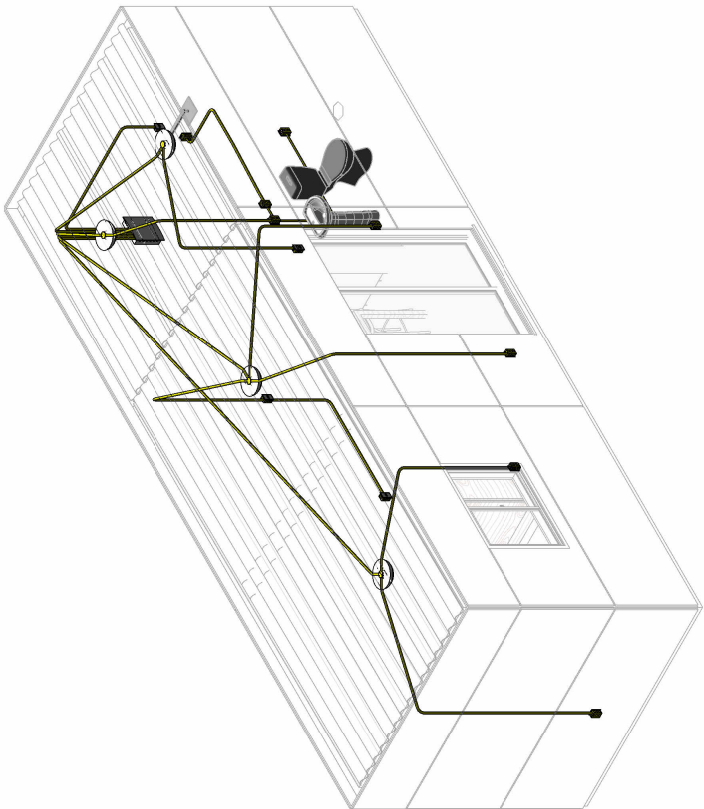
Perspectiva Isométrica
