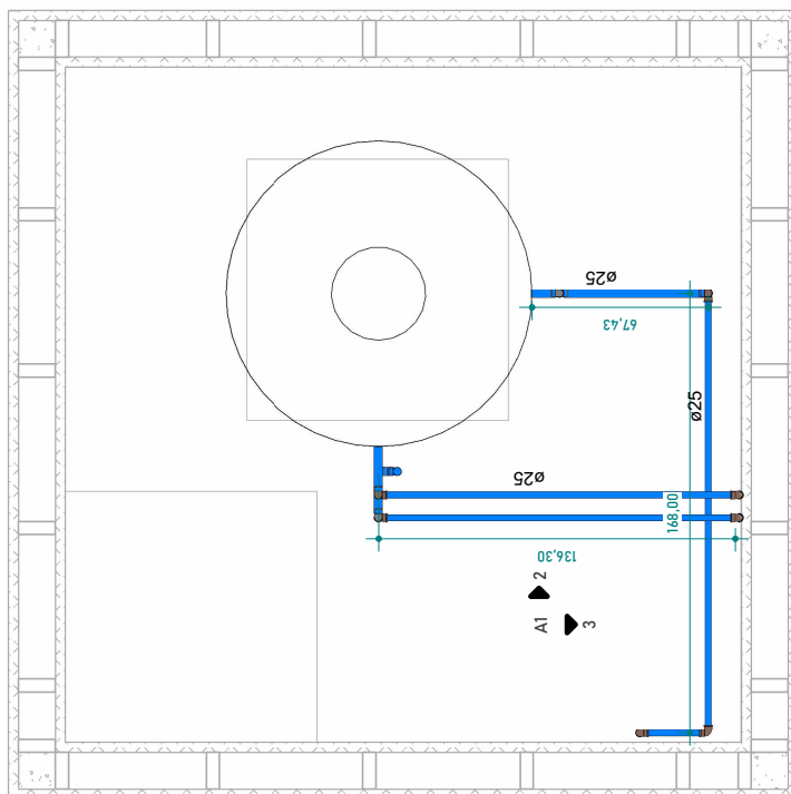
PLANTA BAIXA ESC: 1:20
