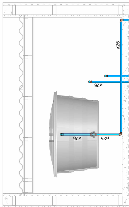
ELE HID - 02 ESC: 1:20
