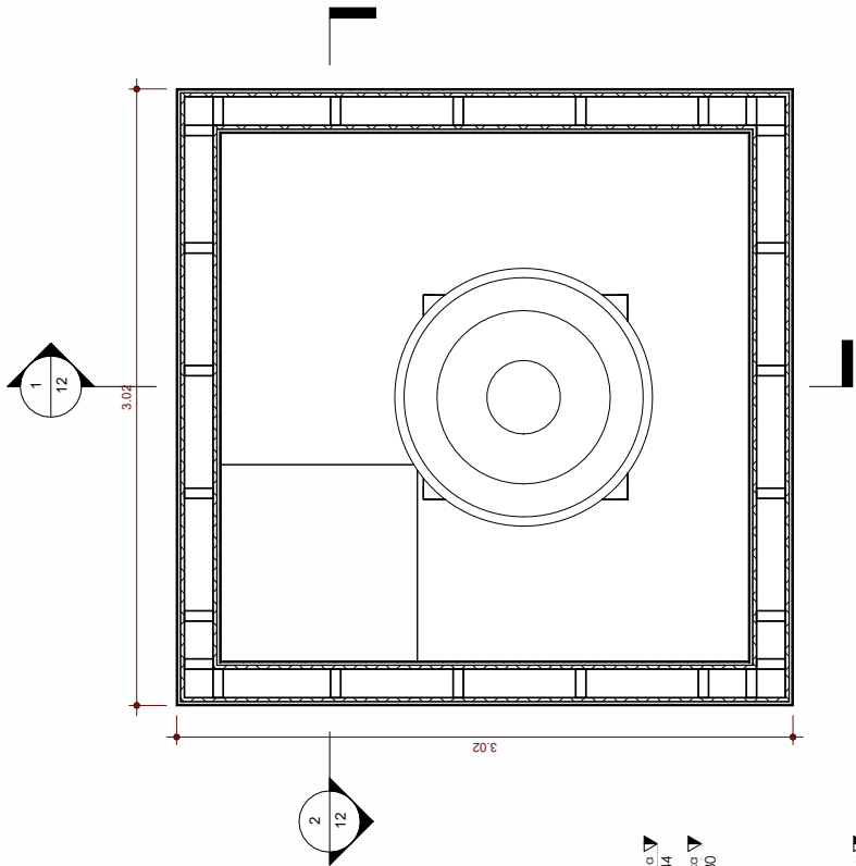
Planta modulo 3x3 - Caixa D'agua ESC: 1 : 25
