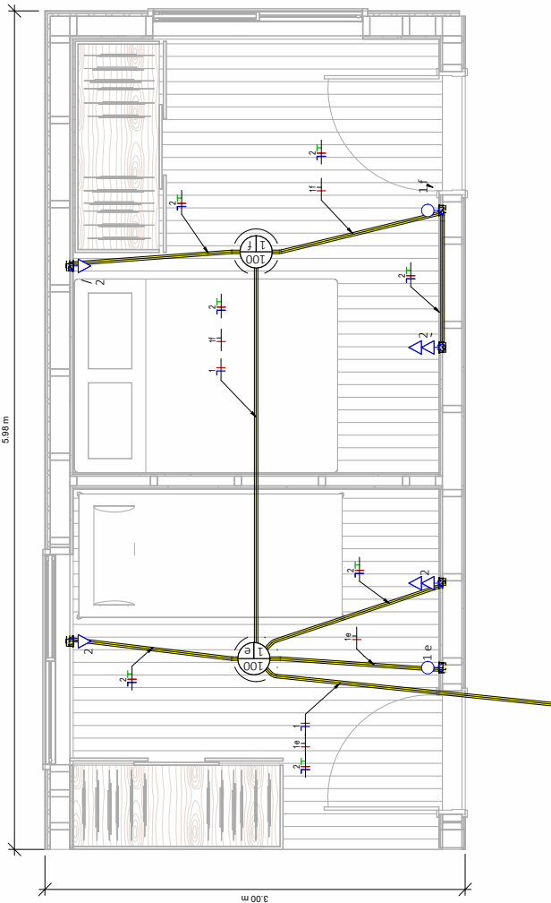
Planta baixa - Elétrica
