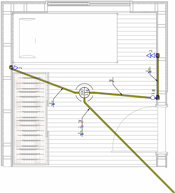
Planta baixa - Elétrica ESC: 1 : 25
