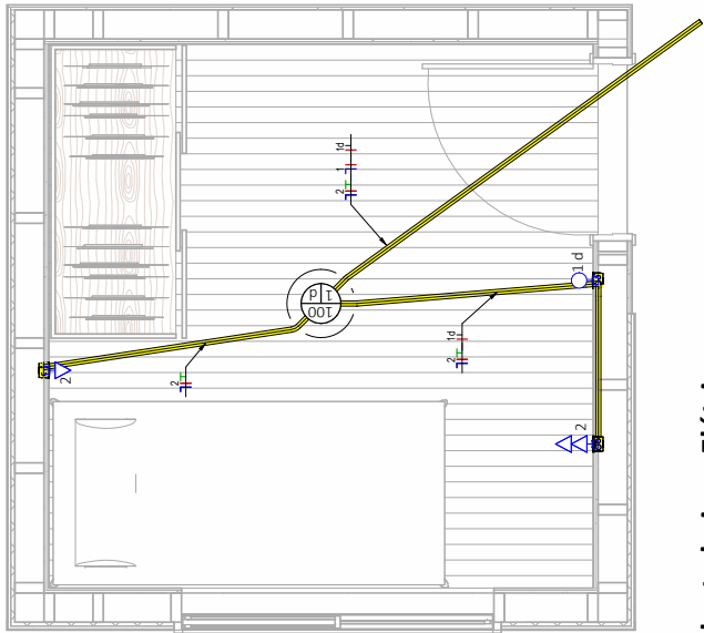
Planta baixa - Elétrica ESC: 1 : 25
