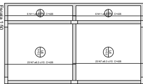
ARMACAO POSITIVA DAS LAJES DO PAVIMENTO PISO RESERVATÓRIOS (EIXO Y)
