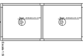
ARMACAO INFERIOR DO RADIER DO PAVIMENTO TERREO (EIXO Y)
