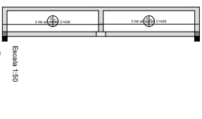
ARMACAO POSITIVA DAS LAJES DO PAVIMENTO COBERTURA (EIXO X)
