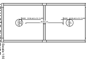
ARMACAO SUPERIOR DO RADIER DO PAVIMENTO TERREO (EIXO Y)
