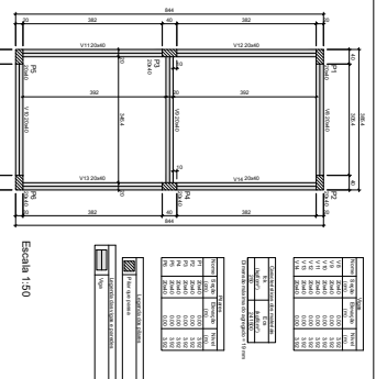
FORMA DO PAVIMENTO VIGAS INTERM (NIVEL 3.92)
