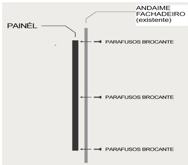
Figura 3: fixação do banner/tapume (já fixado na estrutura de metalon) no andaime fachadeiro existente.
