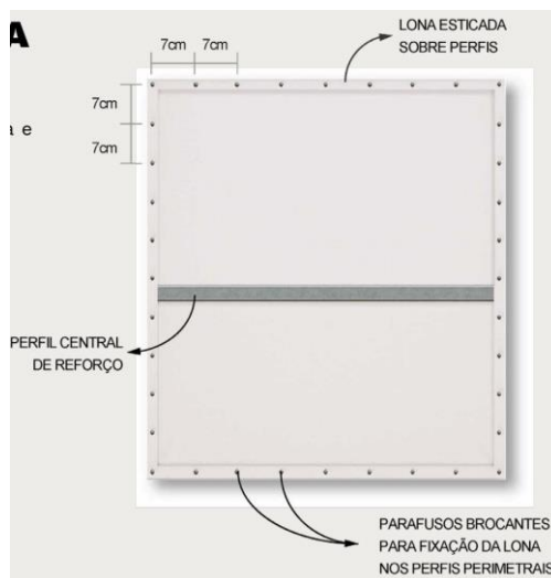
Figura 1: fixação da lona na estrutura de metalon
