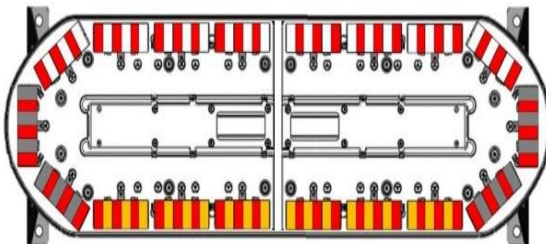
FIGURA 1 - LAYOUT SUGERIDO
