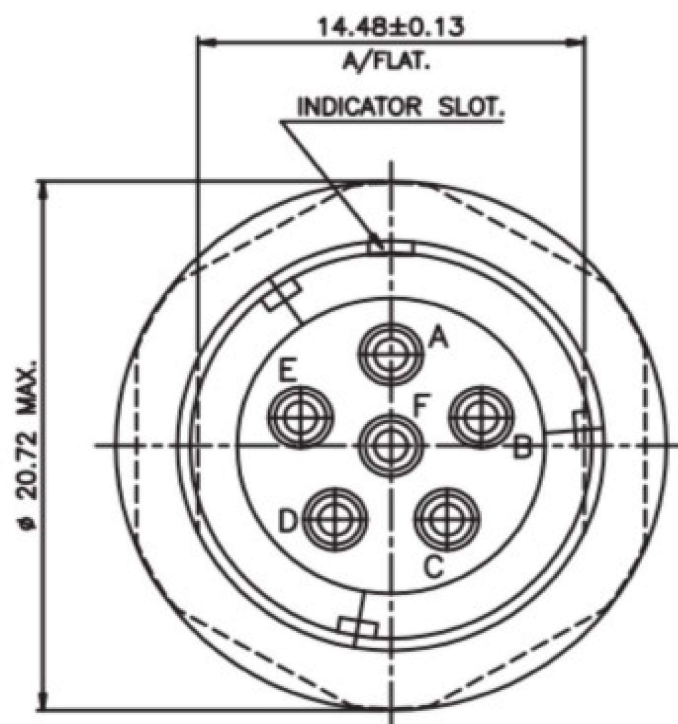
Figura 4-1 Variante de conector de 6 pinos da série Amphenol 164
