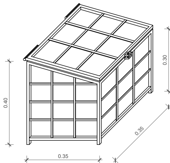
DETALHE - ABRIGO REFLETORES ESCALA 1 / 10
