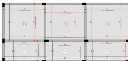
2 Armadura Positiva 1 : 50
