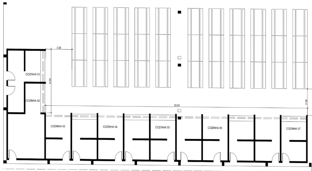
1. PLANTA BAIXA COZINHAS
