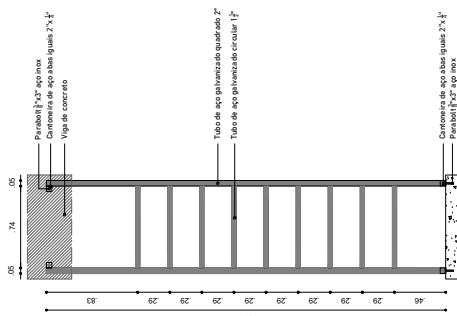
VISTA AA ESC: 1/50
