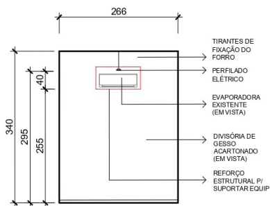
3 VISTA FRONTAL ESCALA 1:50
