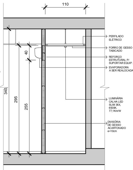
2 CORTE ESCALA 1:25
