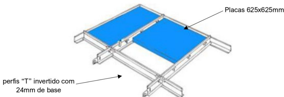
Figura 1: Sistema de fixação do forro modular
