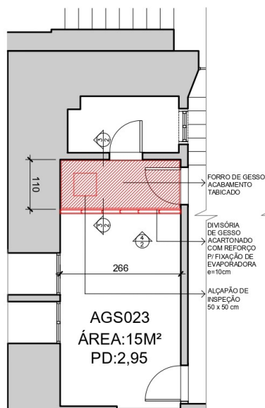
1 PLANTA BAIXA ESCALA 1:50
