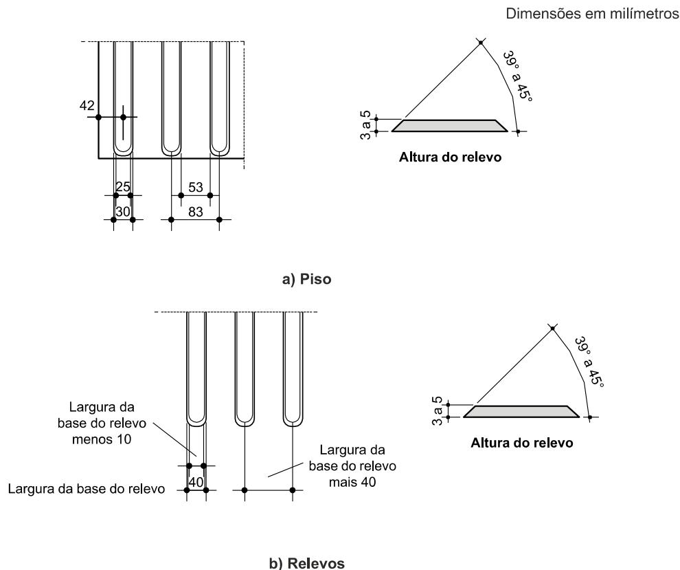
Figura 131 – Sinalização tátil direcional e relevos táteis direcionais instalados no piso
