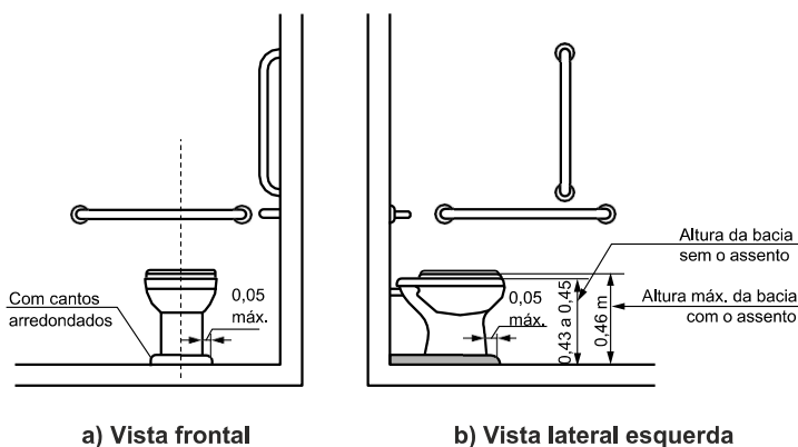
Figura 121– Bacia com sóculo
