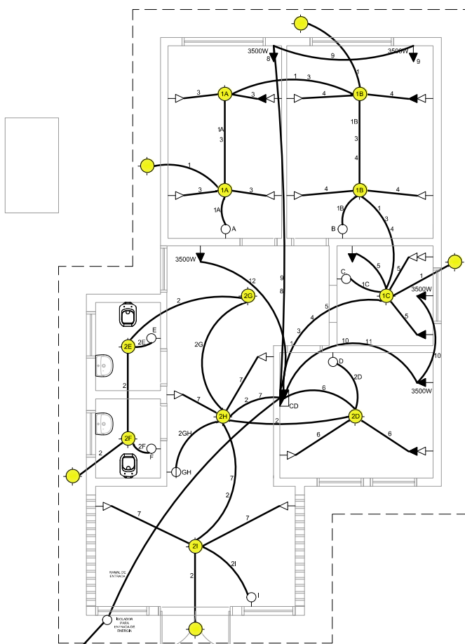
PLANTA BAIXA ELÉTRICA ESC: 1/100
