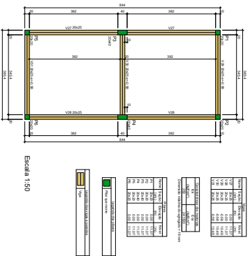
FORMA DO PAVIMENTO PLATIBANDA (NÍVEL 11.07)
