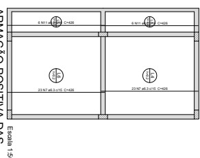
ARMACÃO INFERIOR DO RÁDIER DO PAVIMENTO TÉRREO (EIXO Y)
