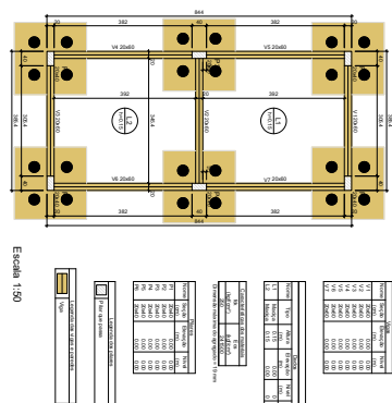
FORMA DO PAVIMENTO TÉRREO (NÍVEL 0.00)
