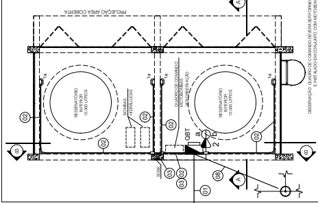
1. ELÉTRICA - PLANTA BAIXA TÉRREO
